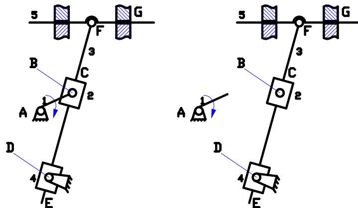
Hình 1-14: Cơ cấu có nhóm loại 3
